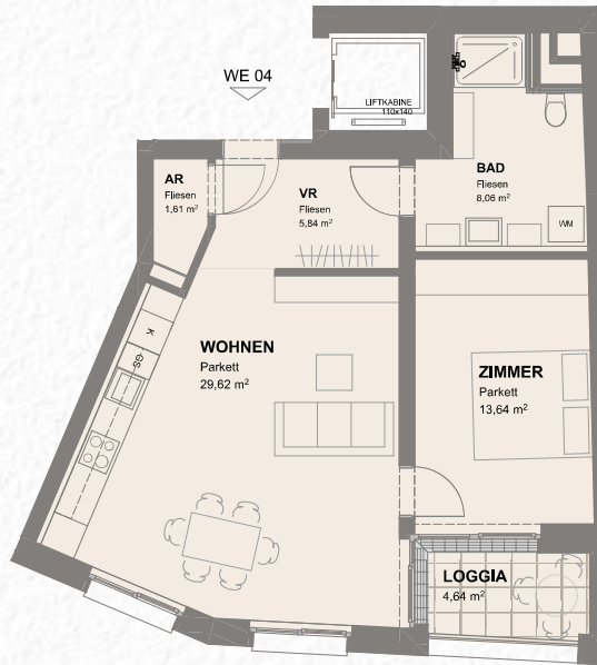
GRUNDRISS TOP 04 – 1:100
