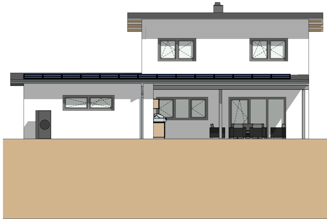
Ansicht SÜDWEST
