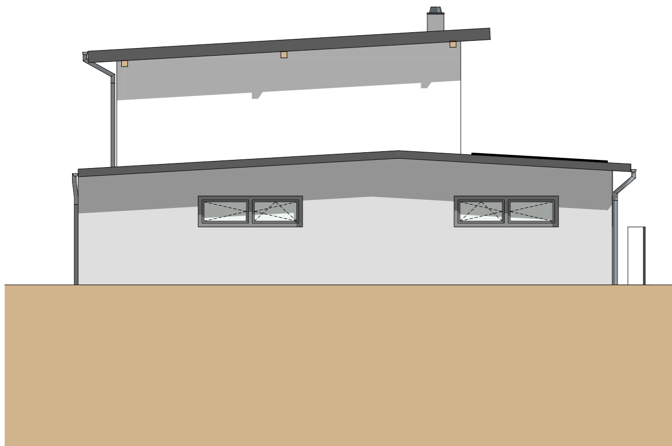
Ansicht NORDWEST
