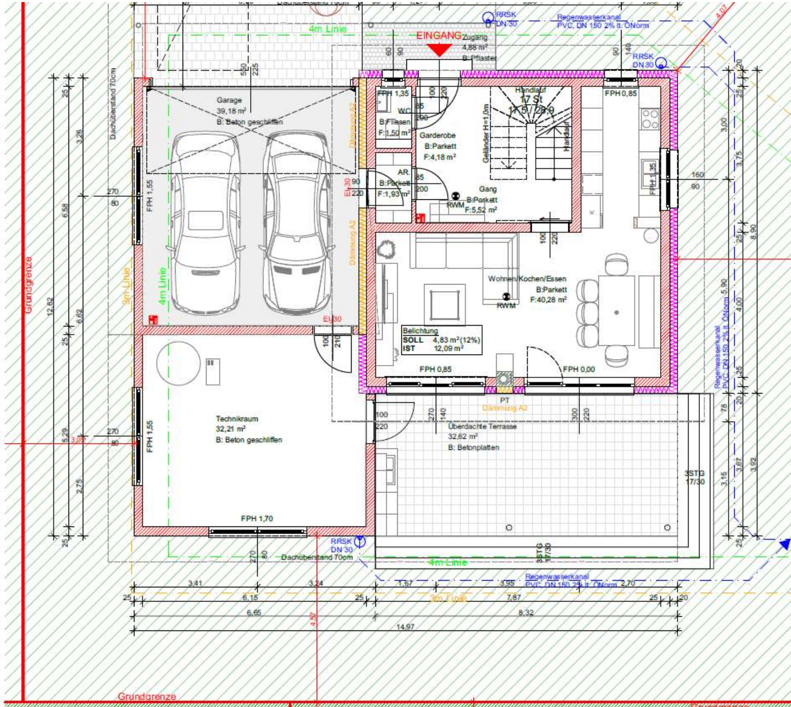
GRUNDRISS EG | M 1:100
