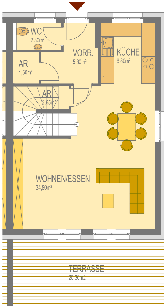
ERDGESCHOSS
